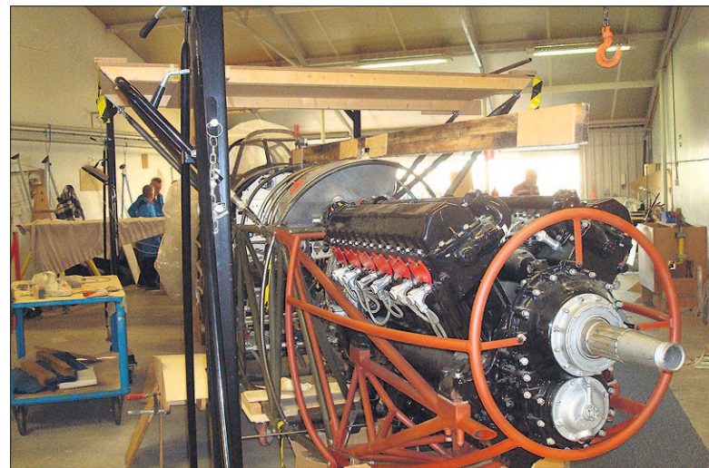
● De overgang van de neus en de romp van de replica in aanbouw van de Fokker C.X die straks een plaats krijgt in het nieuwe Nationaal Militaire Museum.
