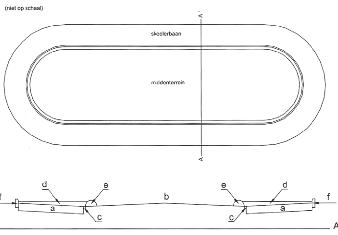
In bovenstaande tekening is een combibaan in zijn meest elementaire vorm weergegeven. In doorsnede A-A is het dwarsprofiel van de combibaan te zien. a = fundering en asfaltlaag, b = middenleren, c = afwateringsgoot, d = ijslaag, e = verharde wal en f = opsluitband
