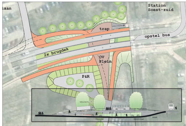
● Bovenaanzicht op het stationsgebied met een OV-passage (schaal 1:500). De inzet toont de verschillende verkeersstromen bij de constructie die de voorkeur heeft van de klankbordgroep. Bron: Klankbordgroep Soest-Zuid
